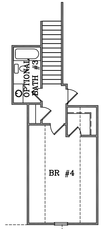
2nd FLOOR PLAN SCALE: N.T.S.
