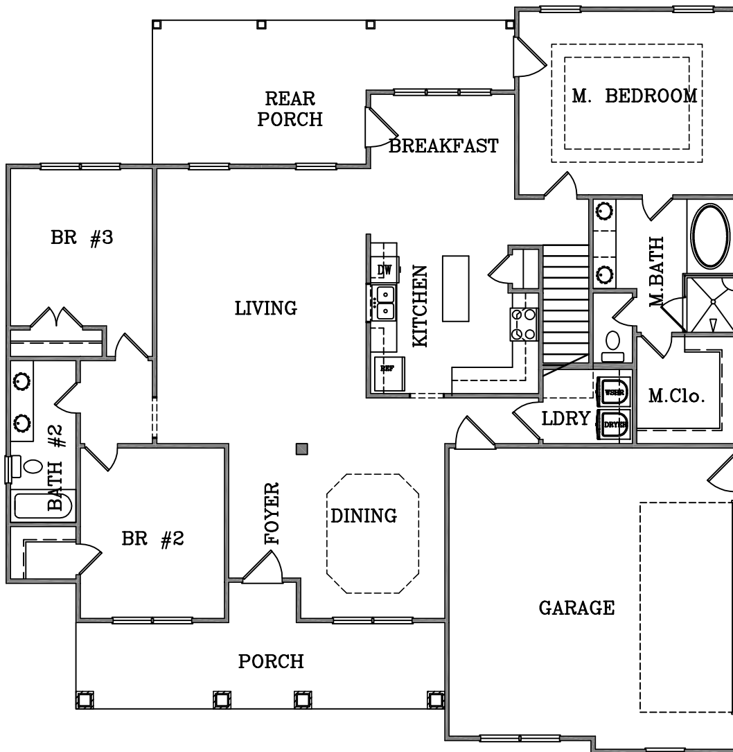
FLOOR PLAN SCALE: N.T.S.
